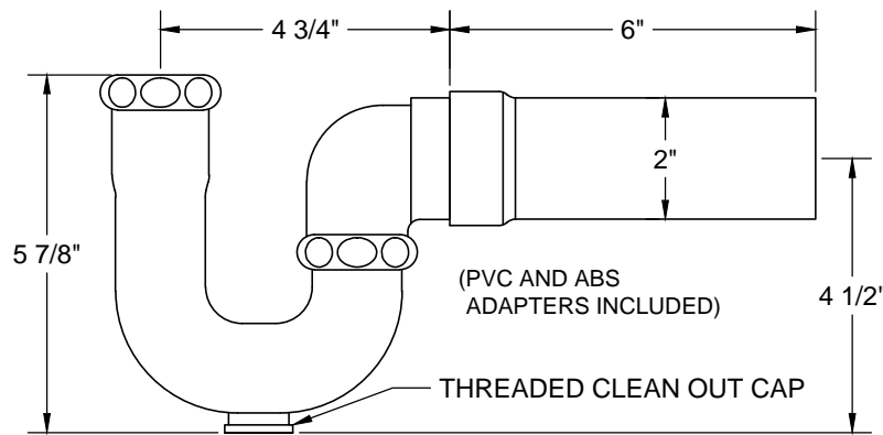
MT304X
