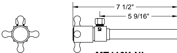
MT416X-NL
